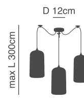
77-8787-243 SE21-SM-19-30-BL3 3xE27, max 60W, 230V
