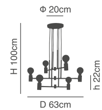
77-8250-160 SE21-BL-100 6xE27, max 60W, 230V
