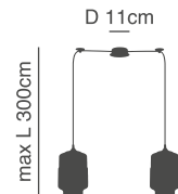
77-8794-139 SE21-HN-18-30-BL2+ 2xE27, max 60W, 230V
