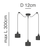
77-8762-105 SE21-BR-B10-BL3-MS1 3xE27, max 60W, 230V
