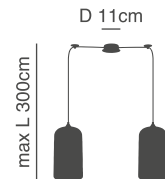
77-8788-165 SE21-SM-19-30-BL2 2xE27, max 60W, 230V
