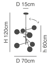
77-4492-202 SE 110-7 7xE14, max 60W, 230V
