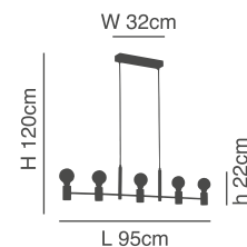
77-8248-145 SE21-NM-120 5xE27, max 60W, 230V
