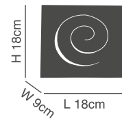
77-1807-41 MX0961-1A 1xG9, max 40W, 230V
