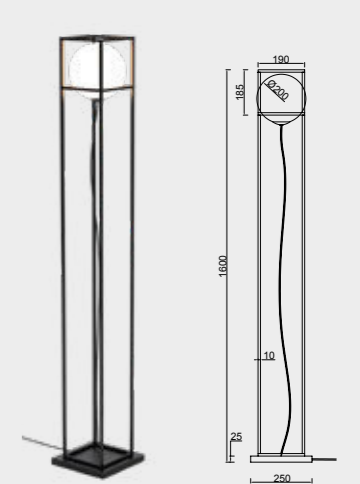
7614 Negro-Black 1LxE27 (no incl)
